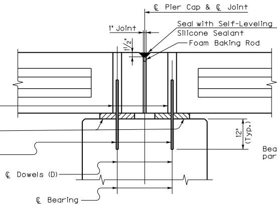
PIER OR PILE BENT
